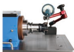
校正刀片公差 Correction insert tolerances
