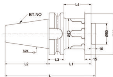
Fig1 标准直柄
