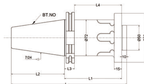
Fig1 标准直柄
