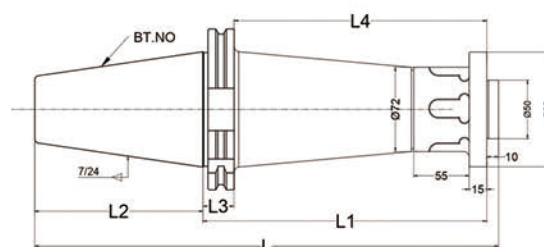
Fig2 加长锥度柄
