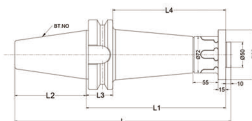
Fig2 加长锥度柄
